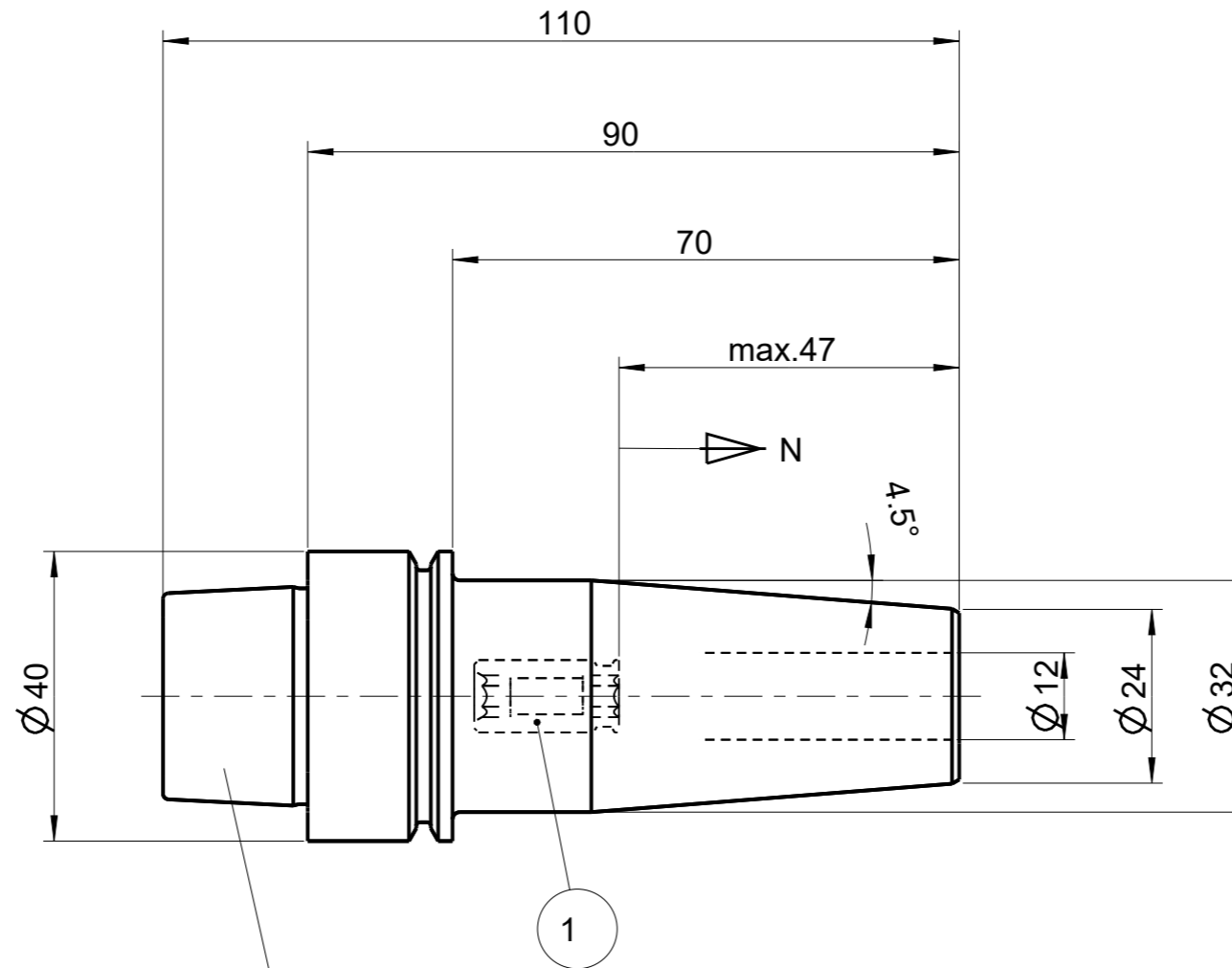
DIN69893-ISO-HSK-E40 mit Anschlussgewinde fuer Kuehlmittelrohr with connection for coolant pipe
