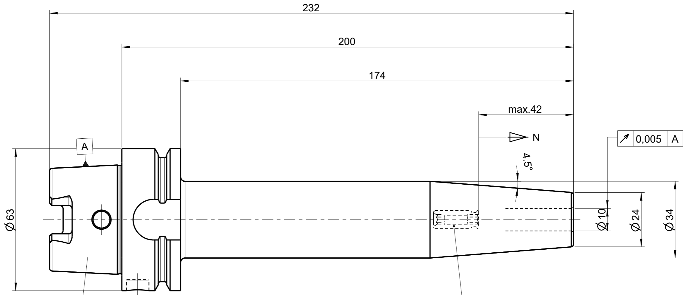
DIN69893-ISO-HSK-A63
